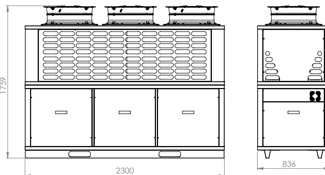
Model osiowy
